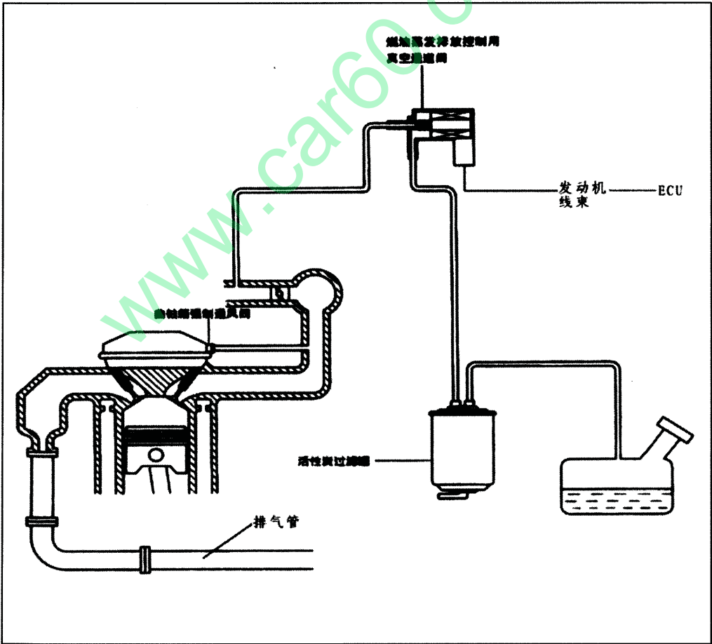
废气排放控制原理图
