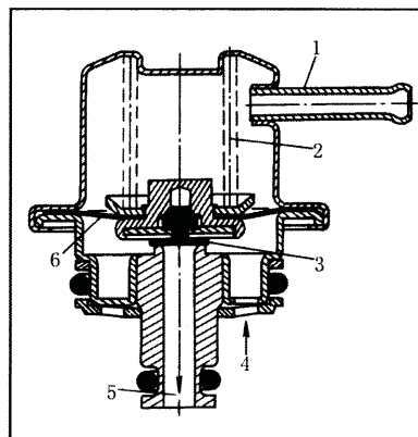
图燃油压力调节器
